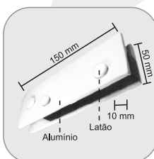
1102 - Zócalo inferior para Pivot Loco (1014)
