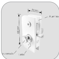
1502 - Cerradura central con rolete
