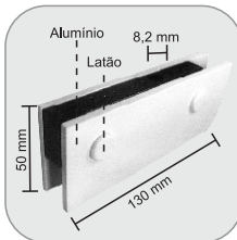
1101 - Zócalo superior - Zamac
