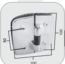
1129-R - D - Bisagra doble automática V/V derecha
