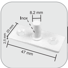
1009 - Buje para Zócalo Superior
