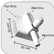
1800C - Passador de Presión
