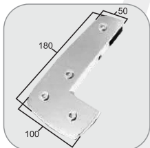
1209-R - Soporte para banderola vidrio / vidrio
