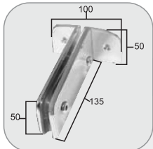
1203-R - Soporte para banderola vidrio / paret
