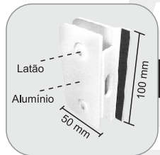
1531 - Contra cerradura central para 1520
