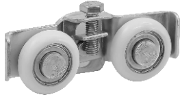
Rueditas Doble con Regulaje CÓD.: 1125D
