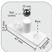
1014 - Pivot loco inferior pivotante
