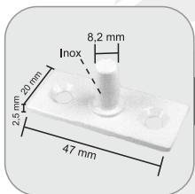
1009 - Buje superior 1101, 1230 e 1231
