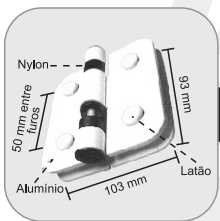
1114 D - Bisagra Doble V/V Aut. - Derecha
