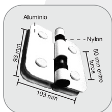
1114 E - Bisagra Doble V/V Aut. - Izquierda
